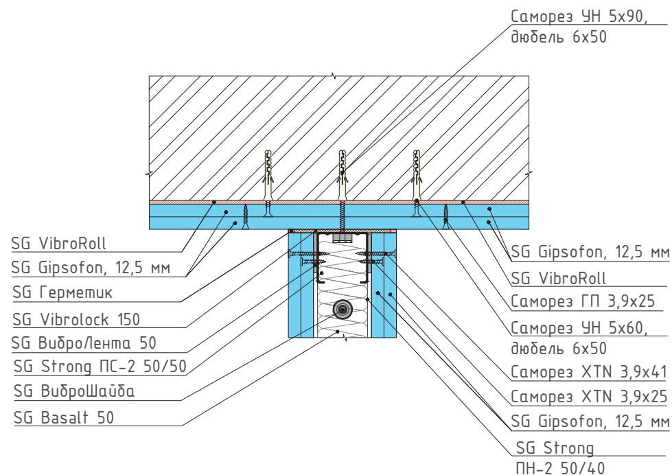
16 Узел примыкания конструкции звукоизоляционной перегородки к бескаркасной системе звукоизоляции стены
