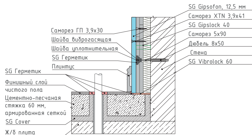
4 Узел сопряжения бескаркасной системы звукоизоляции стены с системой звукоизоляции пола под стяжку
