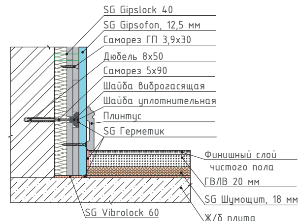
2 Узел сопряжения бескаркасной системы звукоизоляции стены с системой звукоизоляции пола под финишное покрытие
