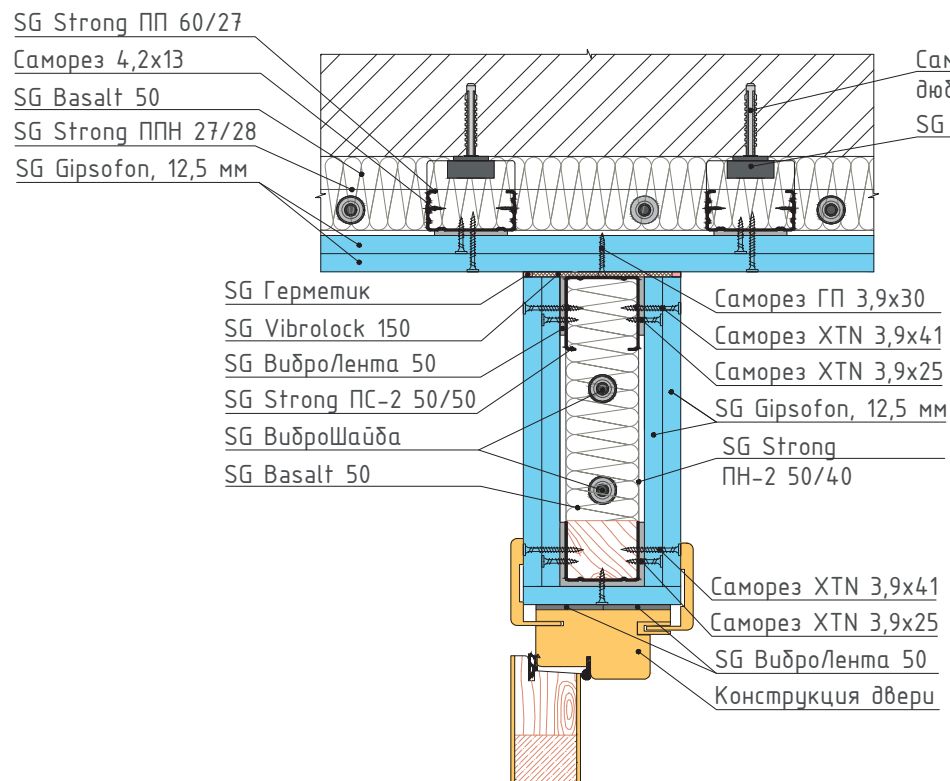
10 Узел примыкания конструкции звукоизоляционной перегородки к каркасной системе звукоизоляции стены
