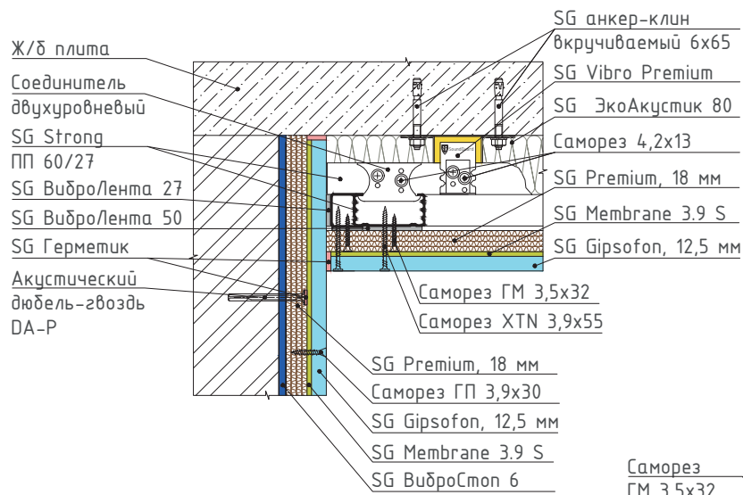
1 Узел сопряжения системы звукоизоляции потолка с бескаркасной системой звукоизоляции стены
