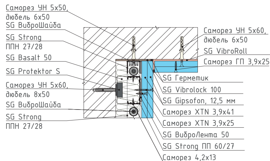
12 Узел сопряжения каркасной системы с бескаркасной системой звукоизоляции стены (внутренний угол)
