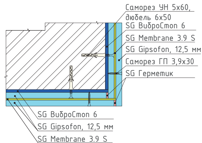
17 Узел сопряжения бескаркасных систем звукоизоляции стен (наружный угол)
