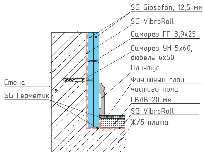
4 Узел сопряжения бескаркасной системы звукоизоляции стены с системой звукоизоляции пола под финишное покрытие
