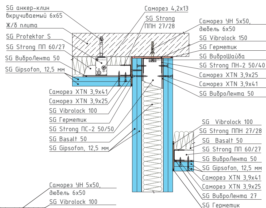
2 Узел сопряжения системы звукоизоляции потолка с конструкцией звукоизоляционной перегородки
