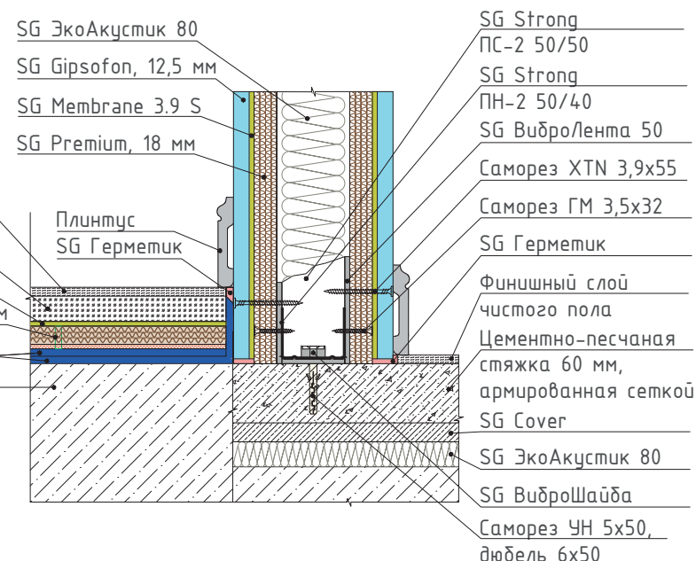
5 Узел сопряжения конструкции звукоизоляционной перегородки с системами звукоизоляции пола под финишное покрытие и пола под стяжку
