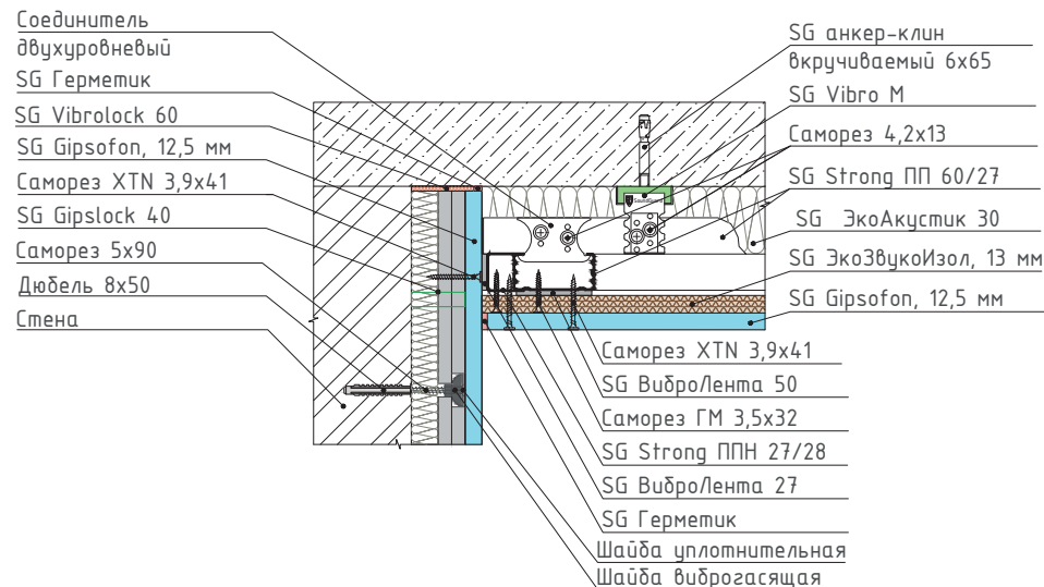
3 Узел сопряжения системы звукоизоляции потолка на откосе с бескаркасной системой звукоизоляции стены
