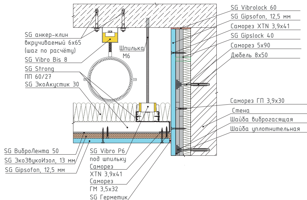
3 Узел сопряжения системы звукоизоляции потолка на откосе с бескаркасной системой звукоизоляции стены
