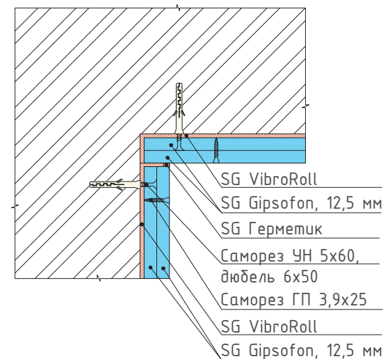
15 Узел примыкания бескаркасной системы звукоизоляции стены к конструкции звукоизоляционной перегородки
